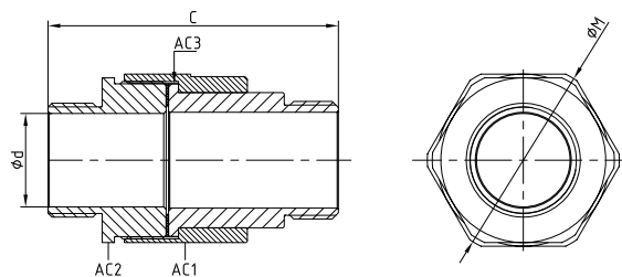
Фитинговые соединения ТСННА, резьба коническая дюймовая NPT
